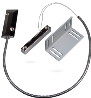
Přejezdový kovový detektor i na kovová vrata s přívodem v pancéřovém krku, 106 x 38 x 10 mm, pracovní vzdálenost max. 75 mm
